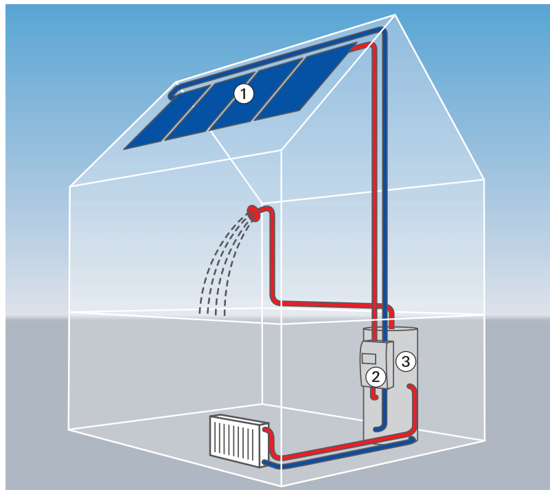
Die wichtigsten Komponenten einer Solaranlage
